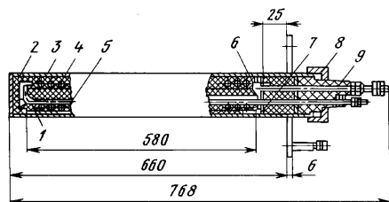
Рис. 1. Габаритные размеры электронагревателя
